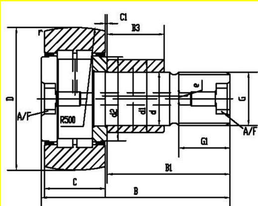
PWKRE... 2RS
