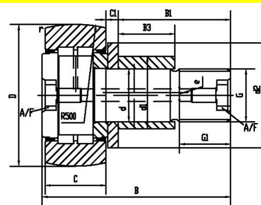
PWKRE35.2RS/PWKRE40.2RS
